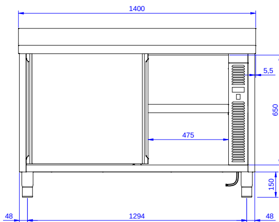
Alzado
